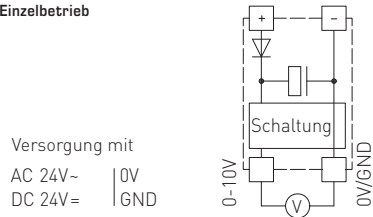
Schaltbild Einzelbetrieb
