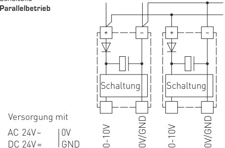
Schaltbild Parallelbetrieb
