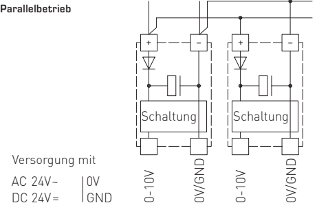
Schaltbild Parallelbetrieb
